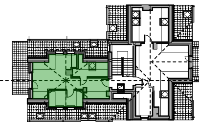
RZUT STRYCHU
